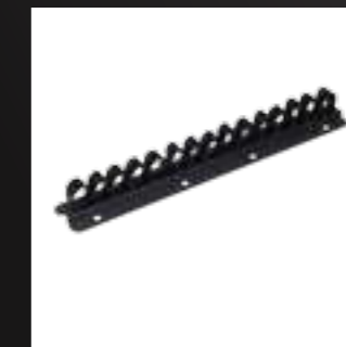
VÆRKTØJSKLEMMELISTE 04-3 WKL 04-3 Art.-nr. 1000003642 Mål: 355 x 33 x 48 mm KR 219,-
